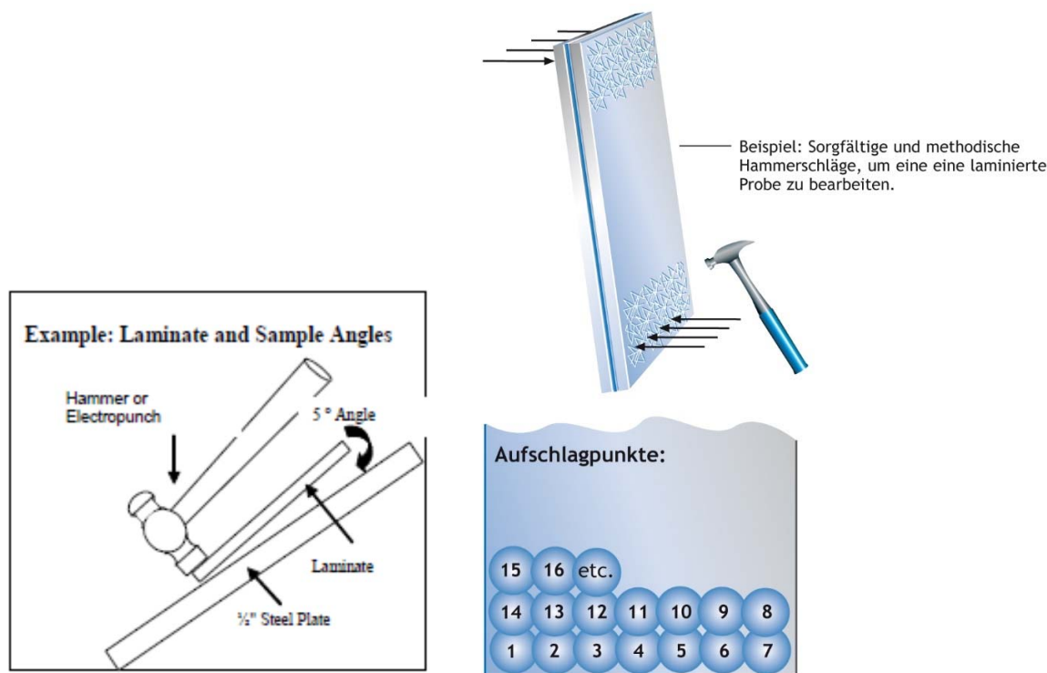
Abb. 3.1: Prüfdurchführung
