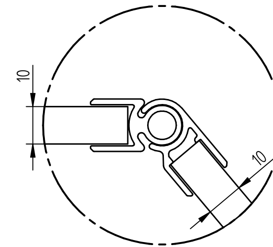
EINZELHEIT A
